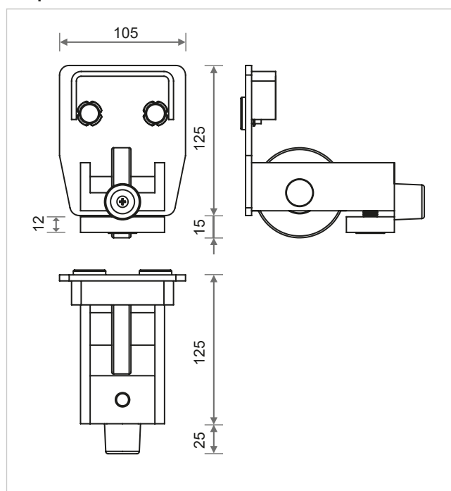
Plaque d'extrémité avec roulement Rollco® LWS 125
