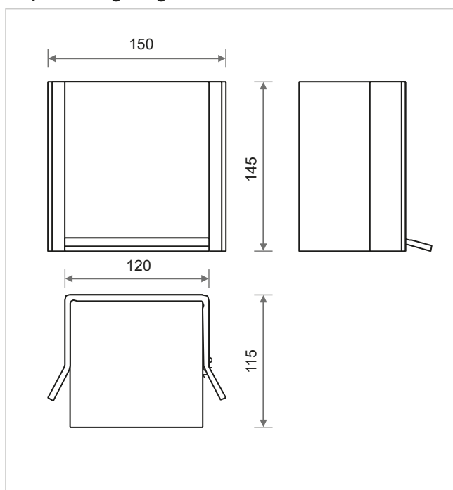
Dispositif de guidage Rollco® LWS 125
