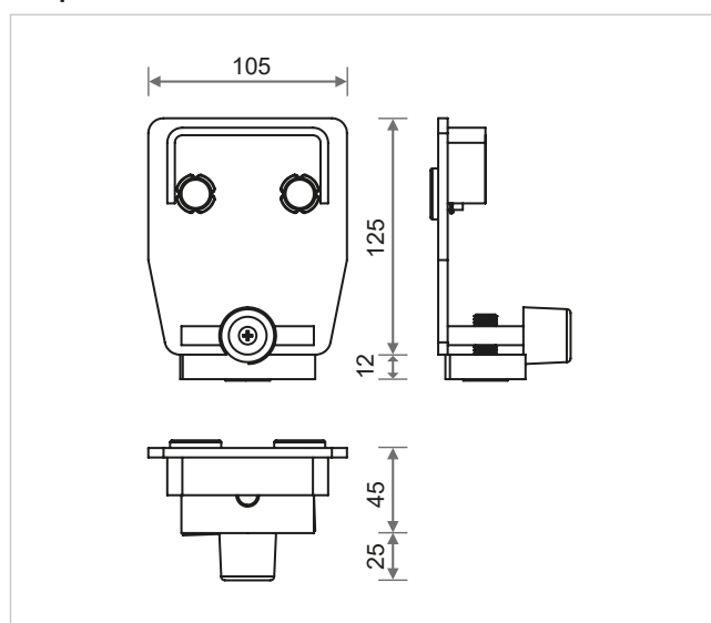
Plaque d'extrémité Rollco® LWS 125
