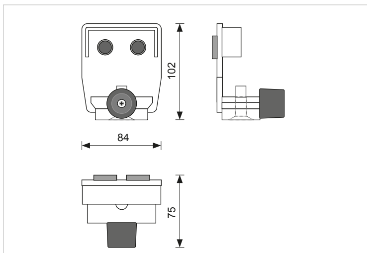
Plaque finale Rollco® LWS 111
