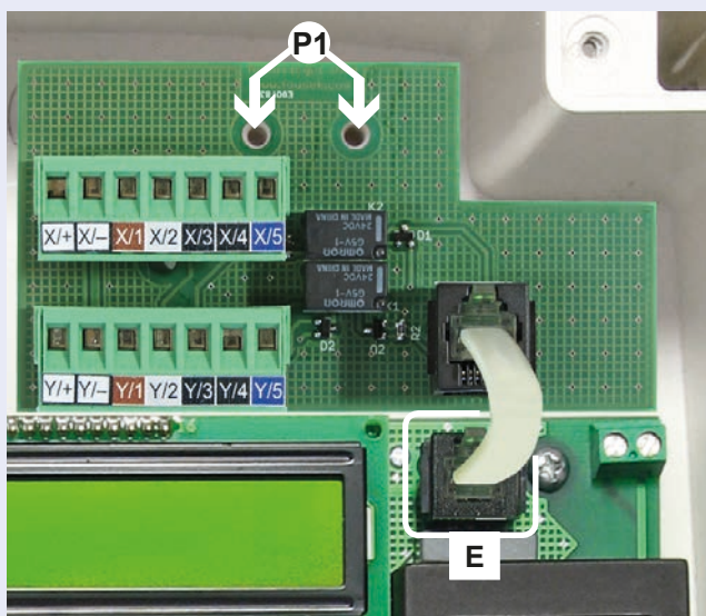
ST REX mit integriertem Motorriegelmodul
