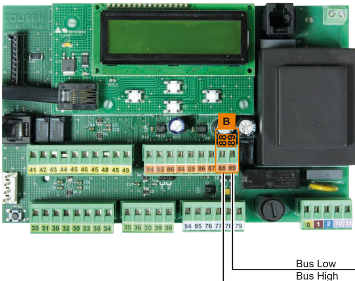
Steuerung ST REX
